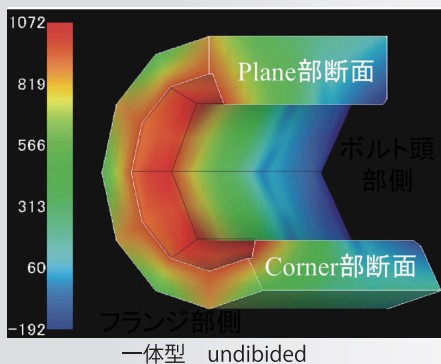
【六角フランジボルト鍛造時のコーナーにかかる応力】
